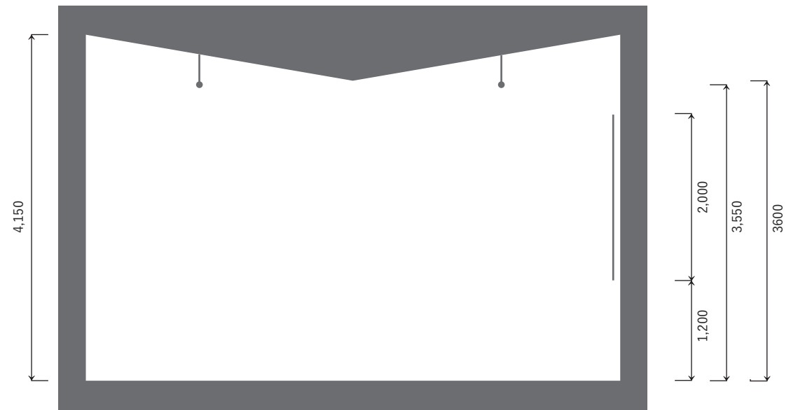
《断面図》
