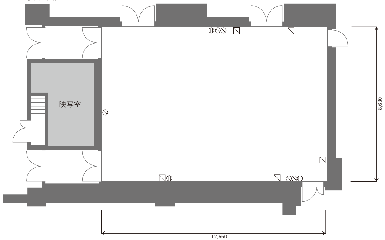
《平面図》
